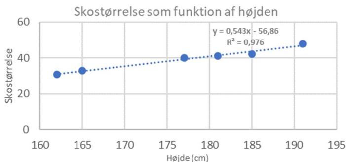
Figur 1: Afbildning af data fra en undersøgelse af sammenhængen mellem skostørrelse og højde for 6 tilfældige testpersoner fra 1.a.
